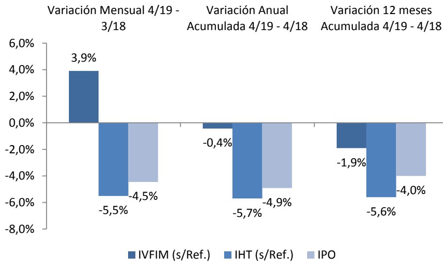
Gráfico 1- Variaciones sin refinería IVFIM, IHT e IPO. Abril 2019
